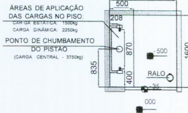
PLANTA BAIXA VIGAS DE POÇO
