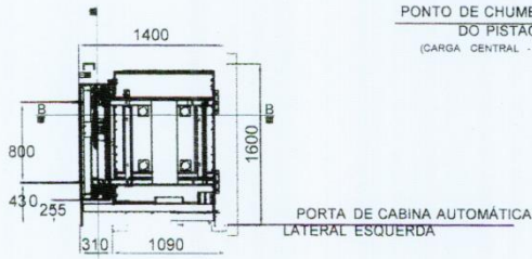
PLANTA BAIXA 1º e 2º PAVIMENTO
